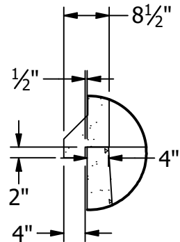
JOINT DETAIL(B) DIMS TYP
