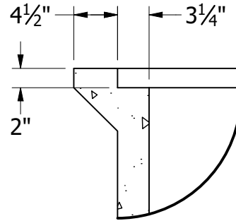
DETAIL B DIMENSIONS TYP
